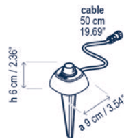
Birdie Base 1 Conexión / Birdie Base 1 Connection
