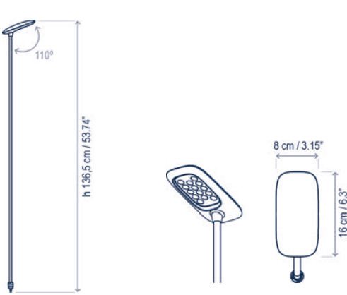
Birdie Luminaria 140L / Birdie Luminaire 140L
