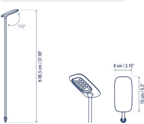
Birdie Luminaria 100L / Birdie Luminaire 100L
