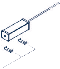
Piezas de fijación para caja de conexión en suelo o pared Fitting set to fix the connection box to the floor or the wall
